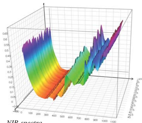
NIR-spectra.
